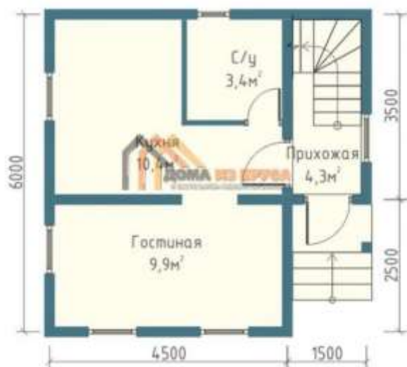
План 1-го этажа
